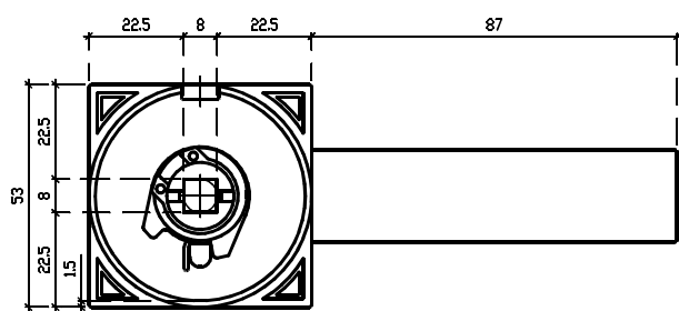
Widok z tyłu klamka I
