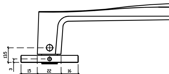
Widok z góry klamka I
