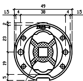
Widok z przodu rozeta montażowa II
