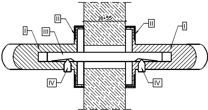
Schemat montażu elementów Przekrój A-A
