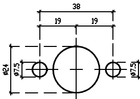
Wymiary otworów montażowych w drzwiach
