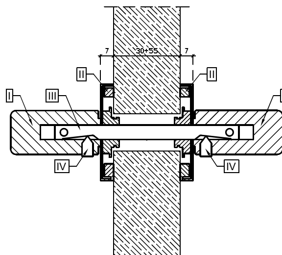
Schemat montażu elementów Przekrój A-A
