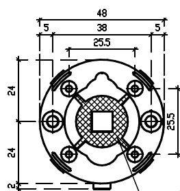
Widok z przodu rozeta montażowa II
