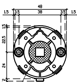
Widok z tyłu rozeta montażowa II
