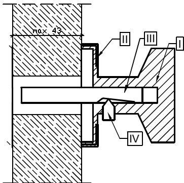
Schemat montażu elementów Przekrój A-A
