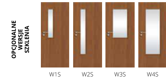
SKRZYDŁA DO OŚCIEŻNICY METALOWEJ str. 222 OŚCIEŻNICA METALOWA str. 226, 228
