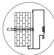
otwór montażowy kotwy w centrum profilu na pierśi ościeżnicy
