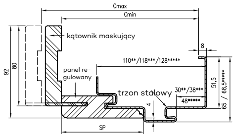
Profil ościeżnicy
