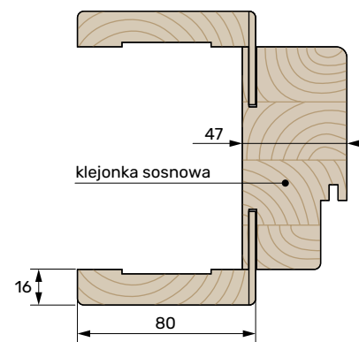
Panel pojedynczy
